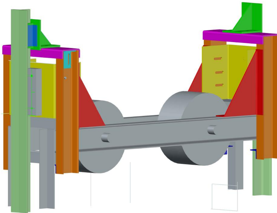
Εικόνα 2: σταθεροποίηση θαλάμου ως προς το σασί (ισομετρικό σχέδιο)
