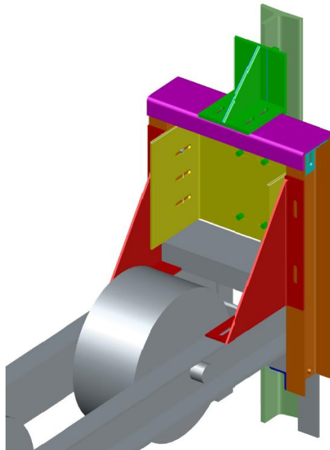
Εικόνα 1. Βάση για στήριξη αρπαγών (ισομετρικό σχέδιο)
